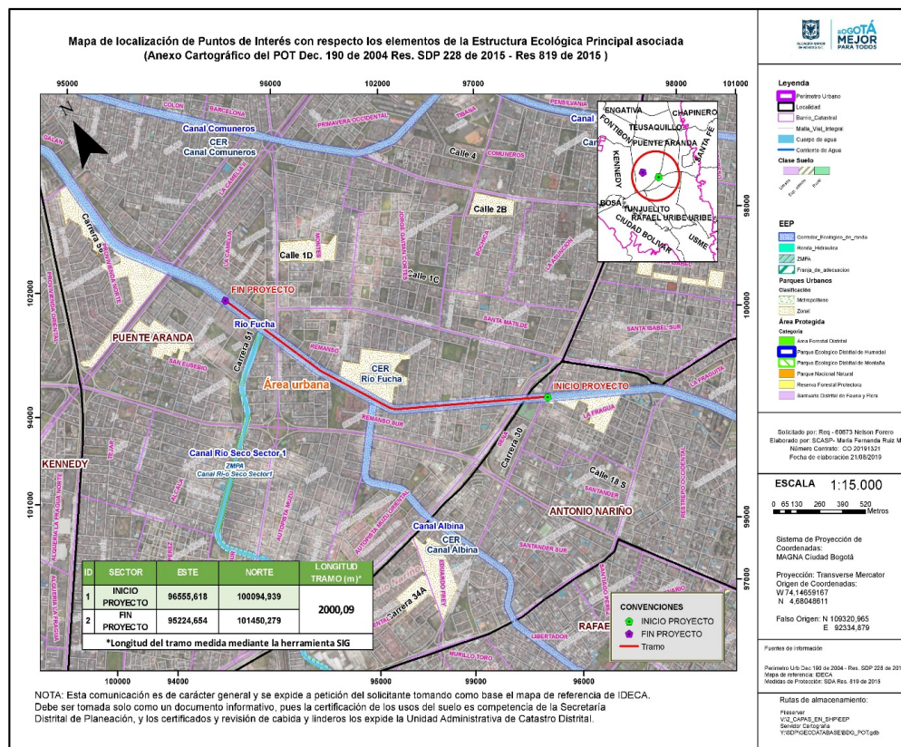
Plano No 1. Localización general del Canal Fucha inicio y final de tramo a intervenir.
